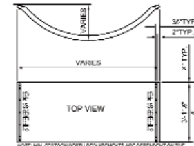
I STIFFENER/GRIPPER DETAIL SCALE: NA
